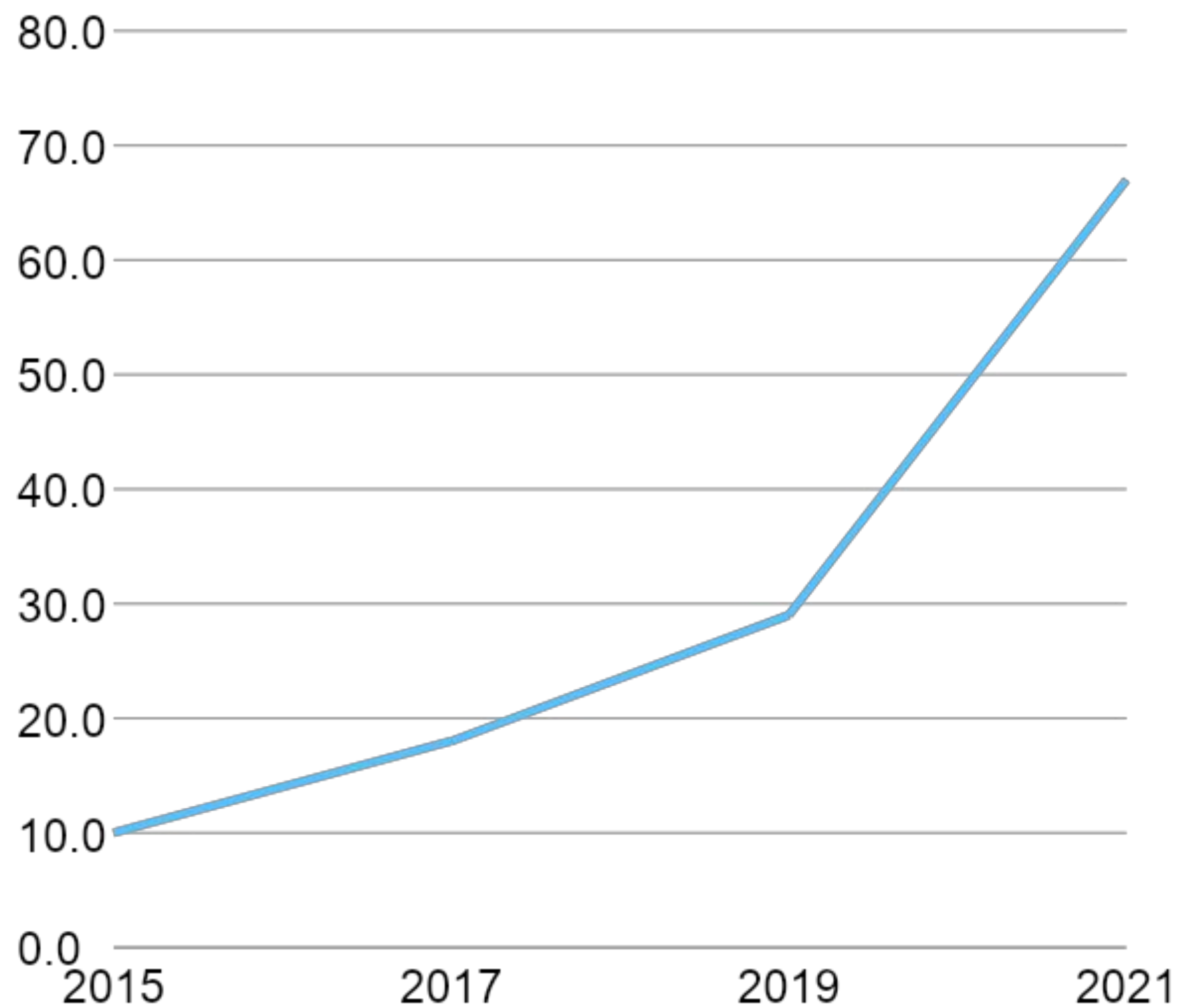
LLMの性能
