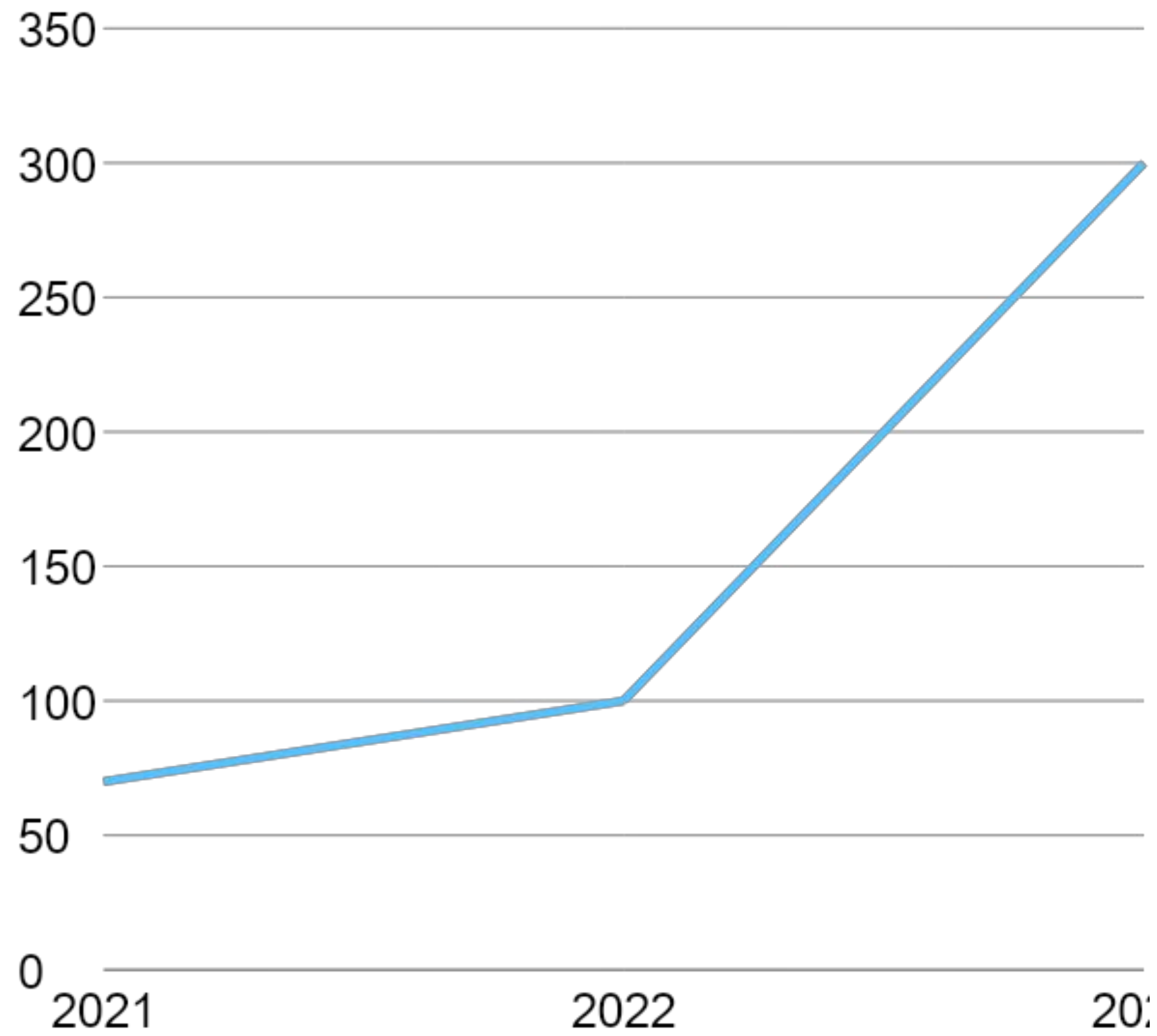
LLMの性能
